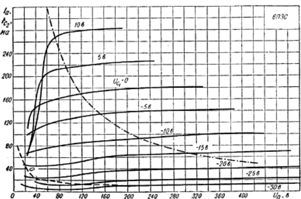
Рис. 391. Усредненные характеристики зависимости тока анода и тока второй сетки от напряжения на второй сетке 250 в: — ток в цепи анода; — — ток в цепи второй сетки; — — наибольшая мощность, рассеиваемая на аноде.
