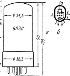
Рис. 387. Лампа 6П3С: а — основные размеры; б — схематическое изображение; 2 и 7 — подогреватель (накал); 3 — анод; 4 — вторая сетка; 5 — первая сетка; 8 — катод.
