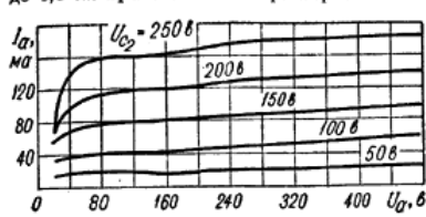
Рис. 390. Усредненные характеристики зависимости тока анода от напряжения на второй сетке 250 в при различных напряжениях на второй сетке и напряжении на первой сетке 0.
