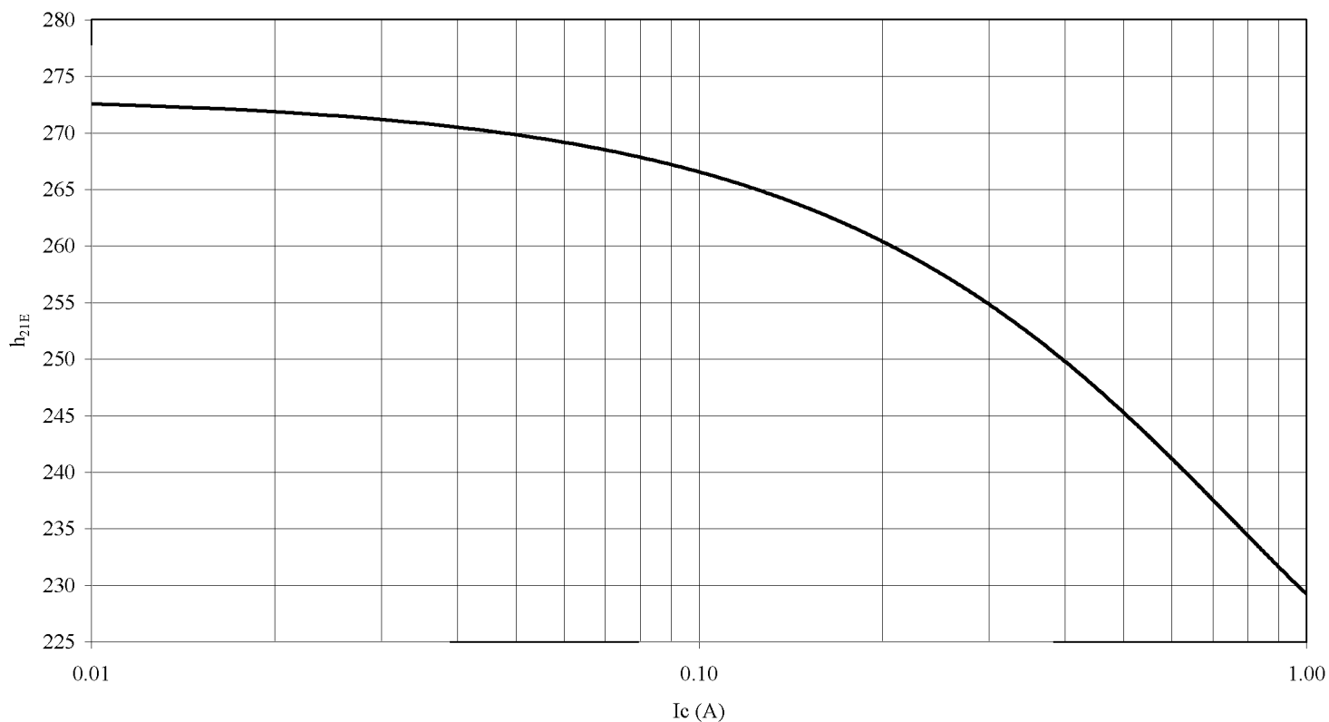
Типовая зависимость h_{21E} = f(I_c) при U_c = 5V , t_{amb} = (25 \pm 10)^\circ\text{C}
