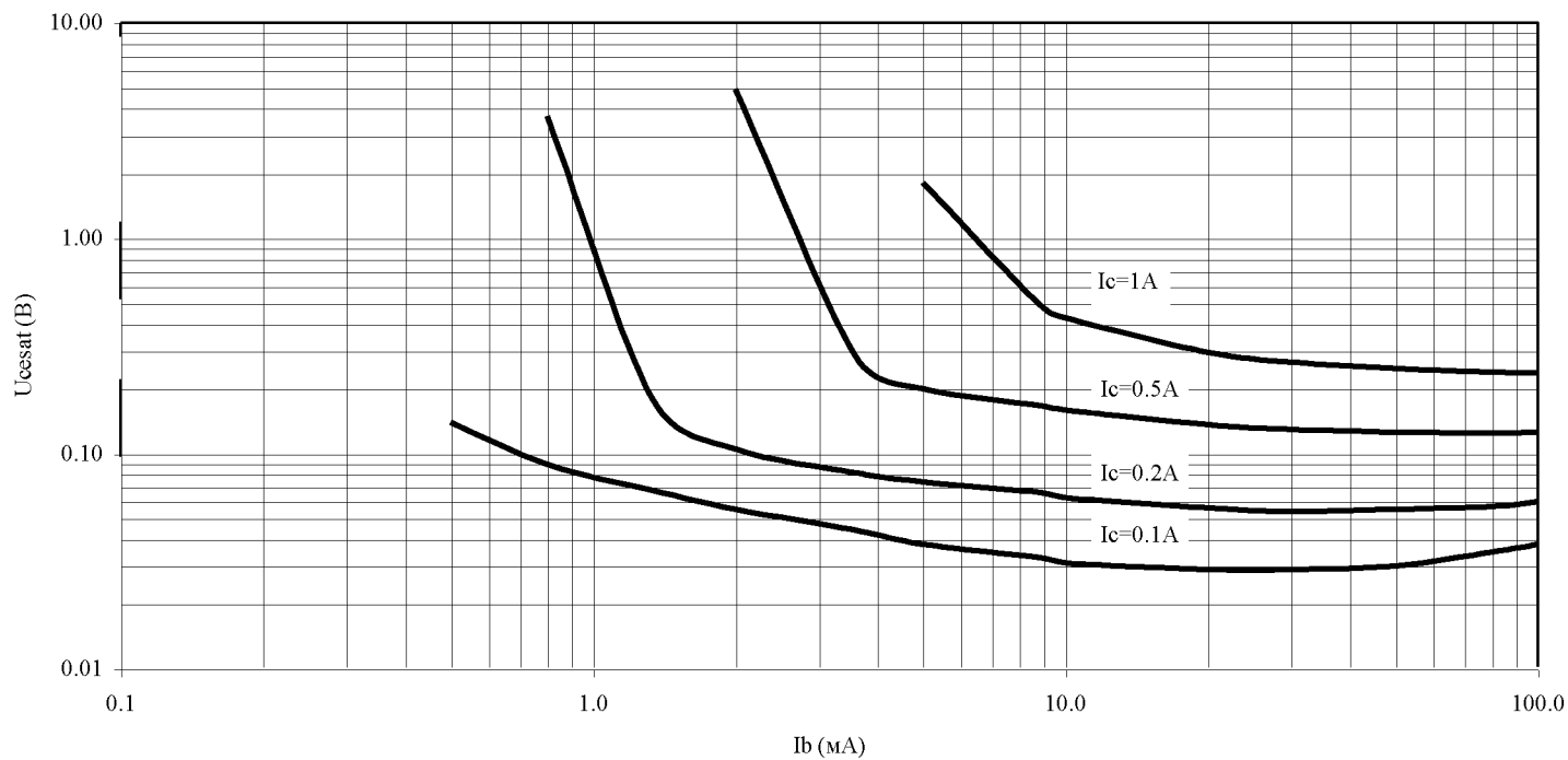
Типовая зависимость U_{cesat} = f(I_b) при t_{amb} = (25 \pm 10)^\circ\text{C}
